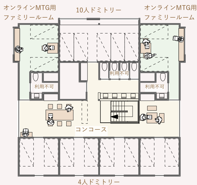
■2階平面図
